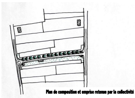
Exemple de schéma d'orientation d'aménagement: voirie travers
