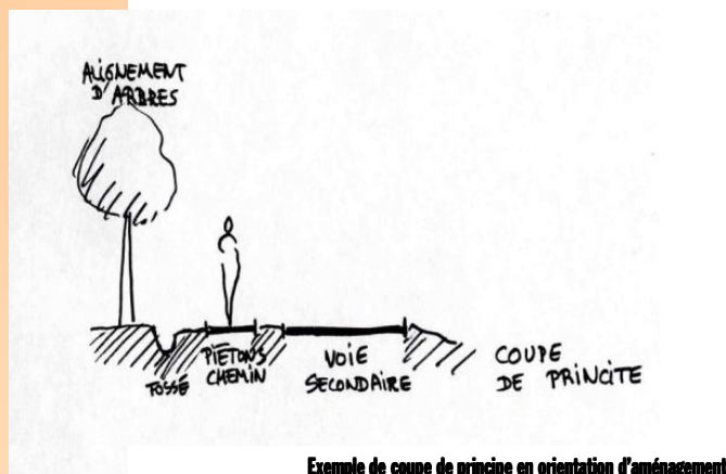
Exemple de coupe de principe en orientation d'aménagement
